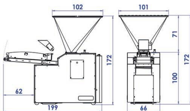
Diviseuse-volumétrique Lofty avec trémie ouverte 200kg
