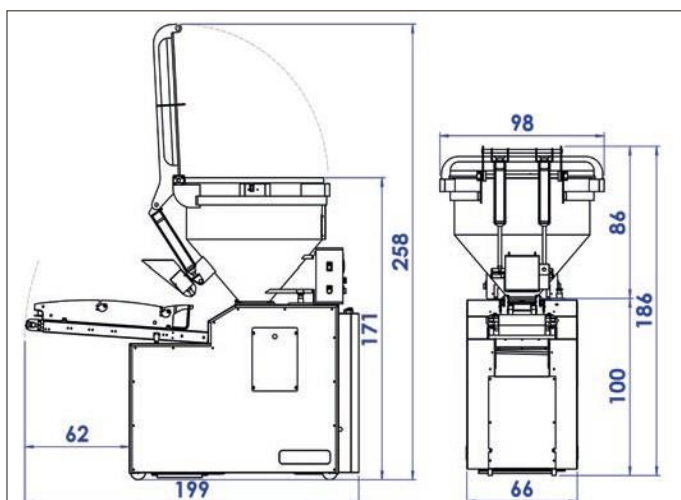
Diviseuse-volumétrique Lofty avec trémie fermée
